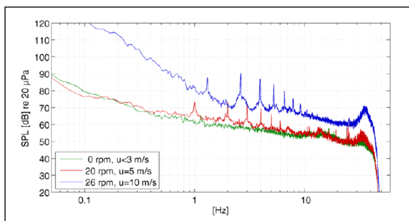
Bild 9: Frequenzanalyse des Schallsignales einer Windkraftanlage bei Hannover
